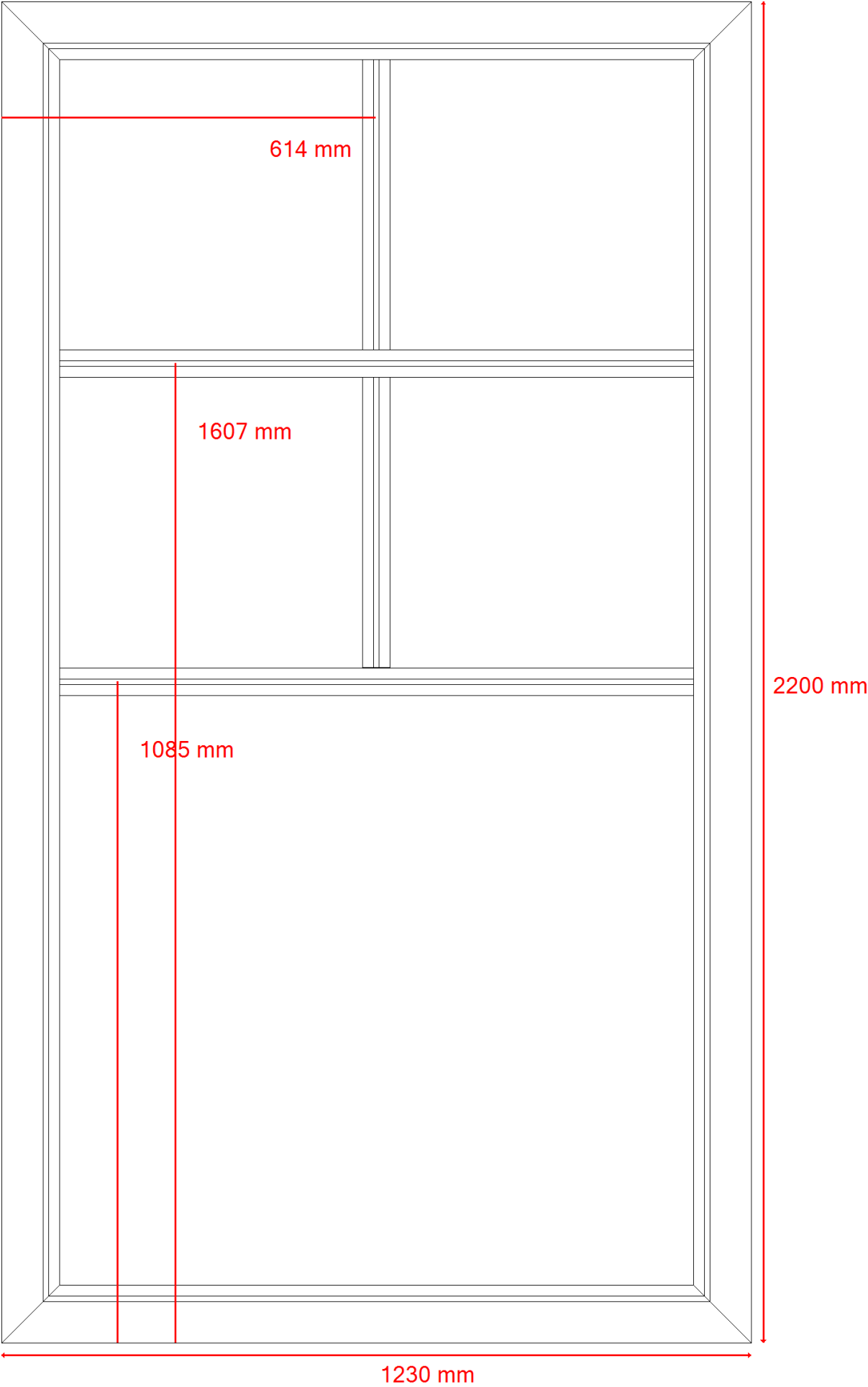
Werktekening incl. bematingen
