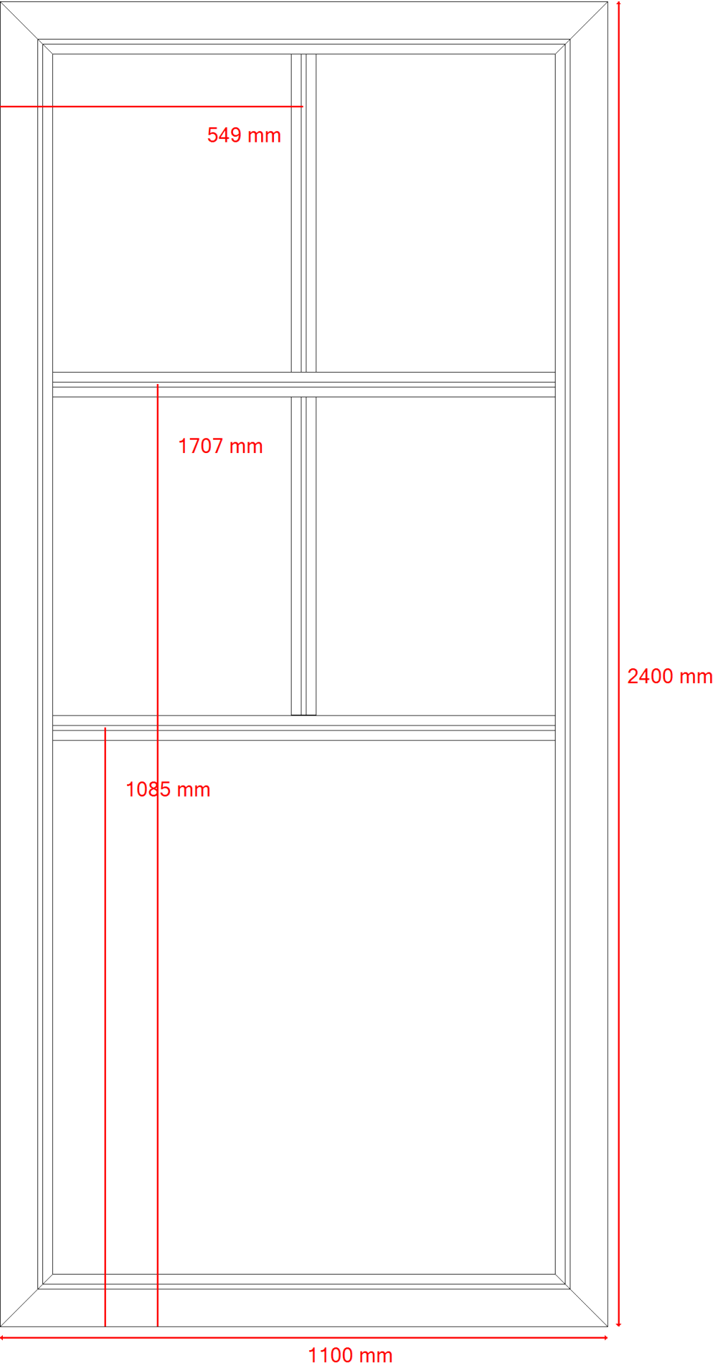
Werktekening incl. bematingen
