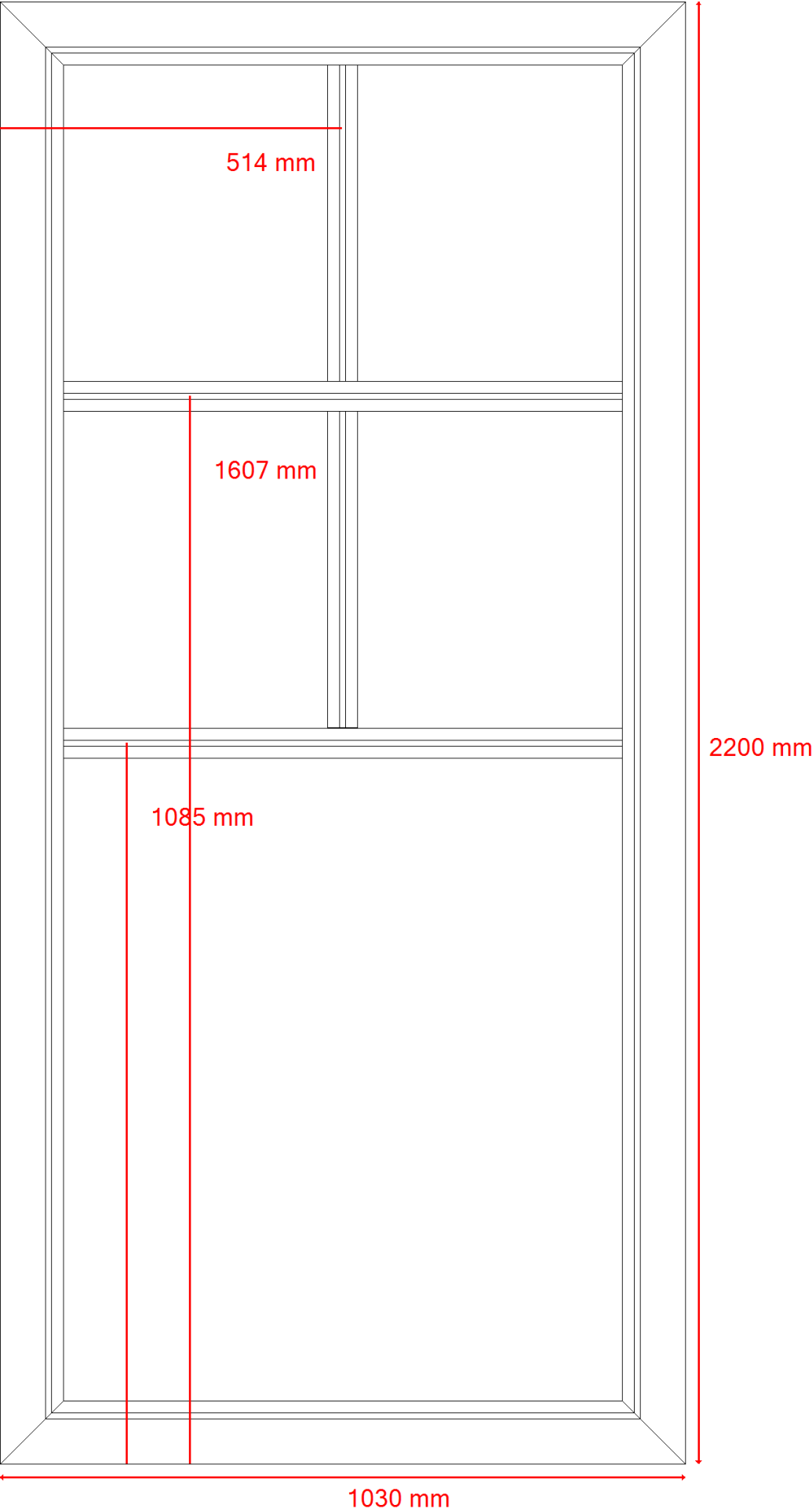
Werktekening incl. bematingen
