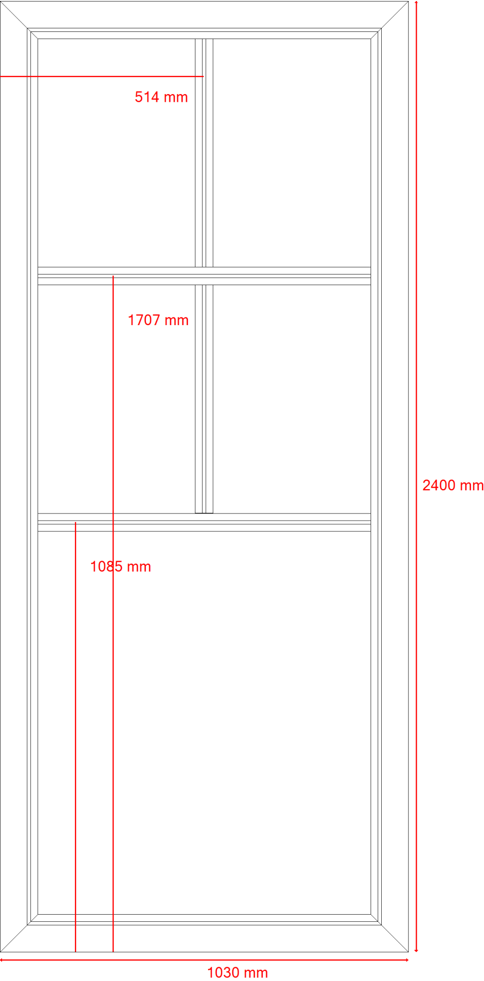
Werktekening incl. bematingen
