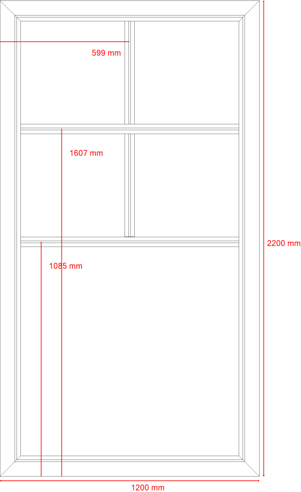
Werktekening incl. bematingen
