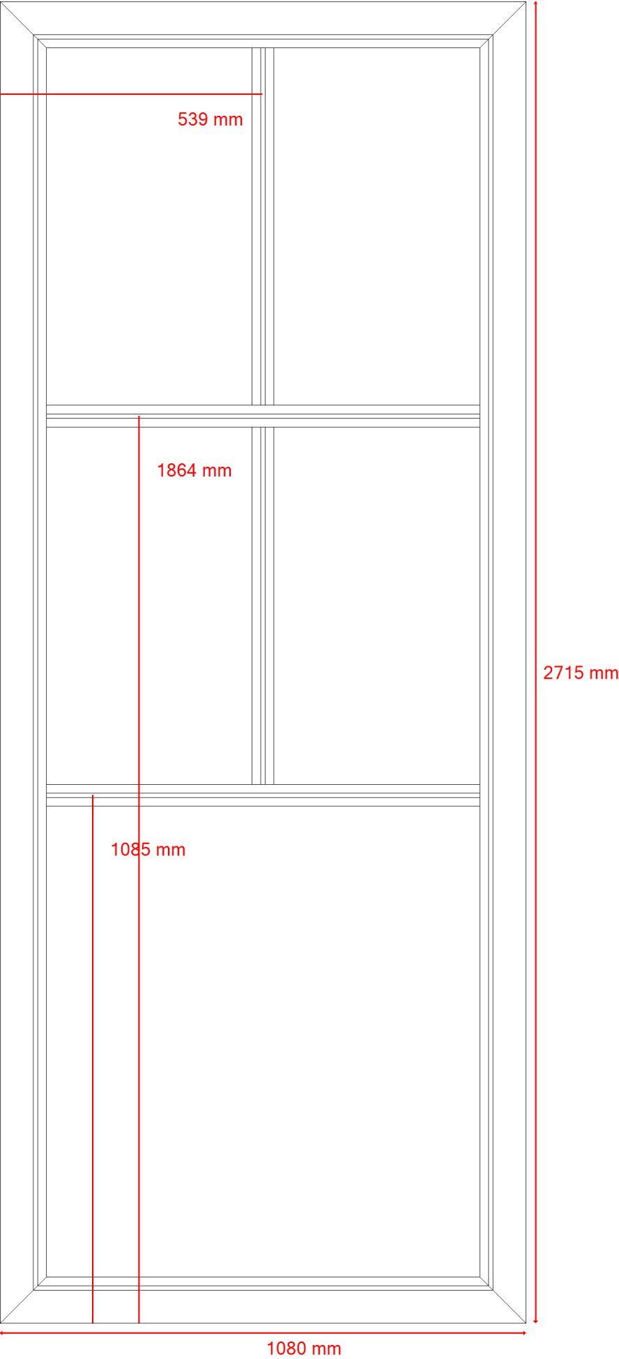
Werktekening incl. bematingen
