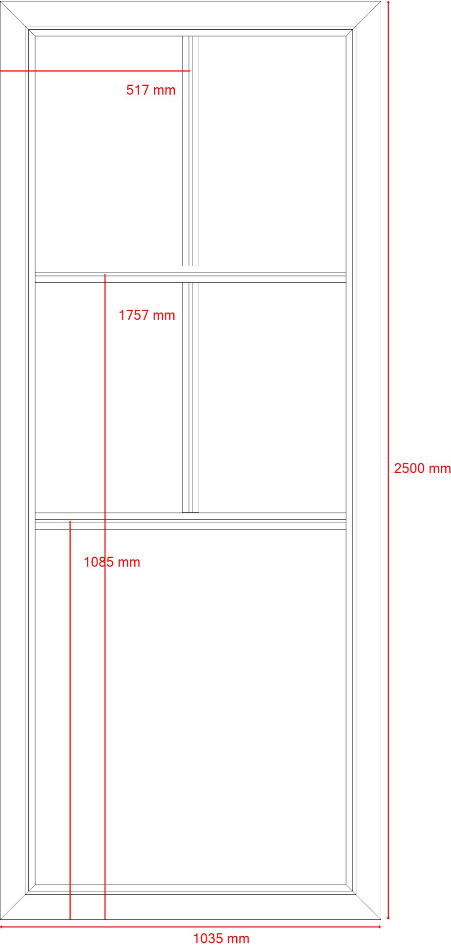
Werktekening incl. bematingen
