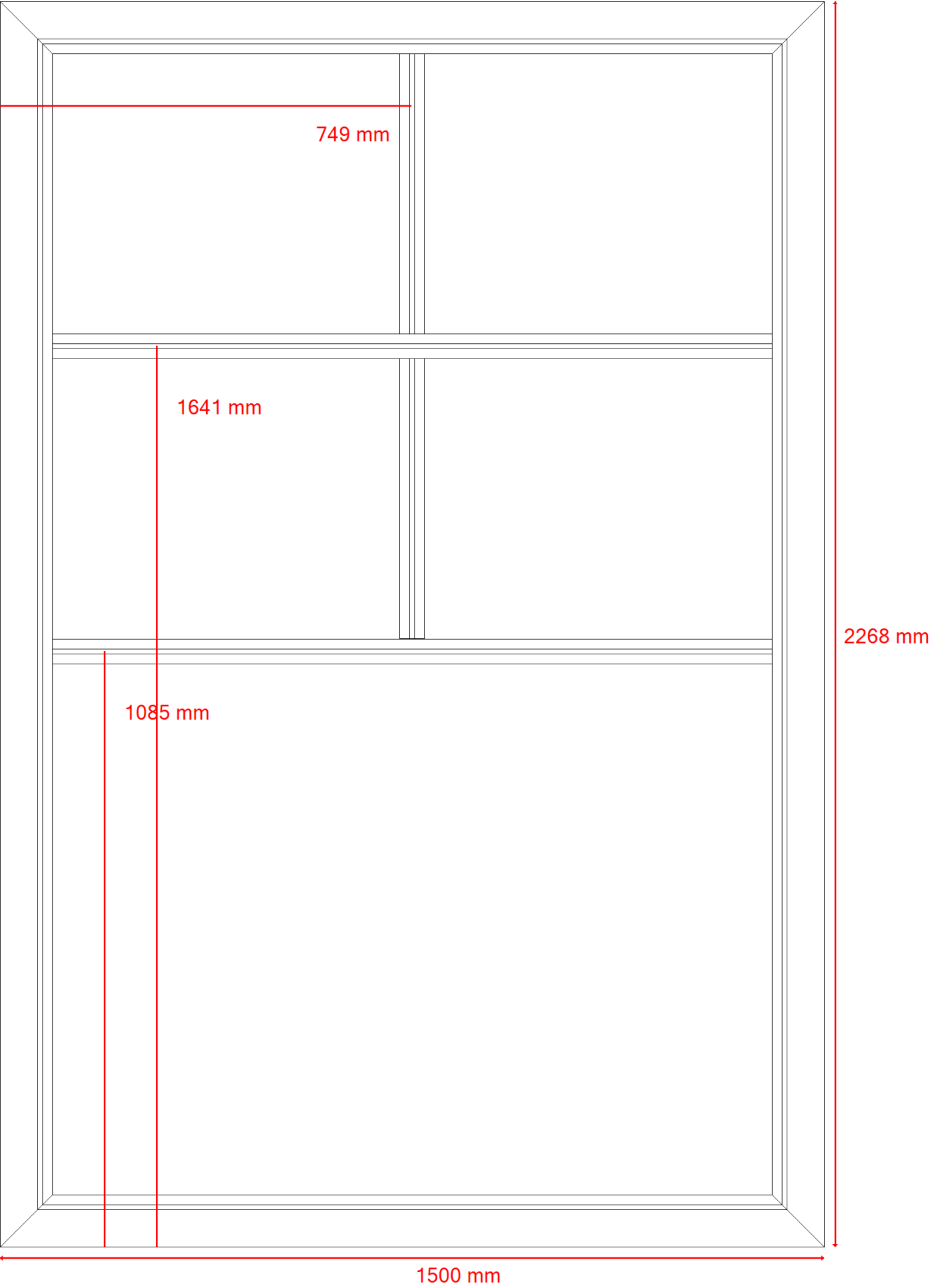
Werktekening incl. bematingen
