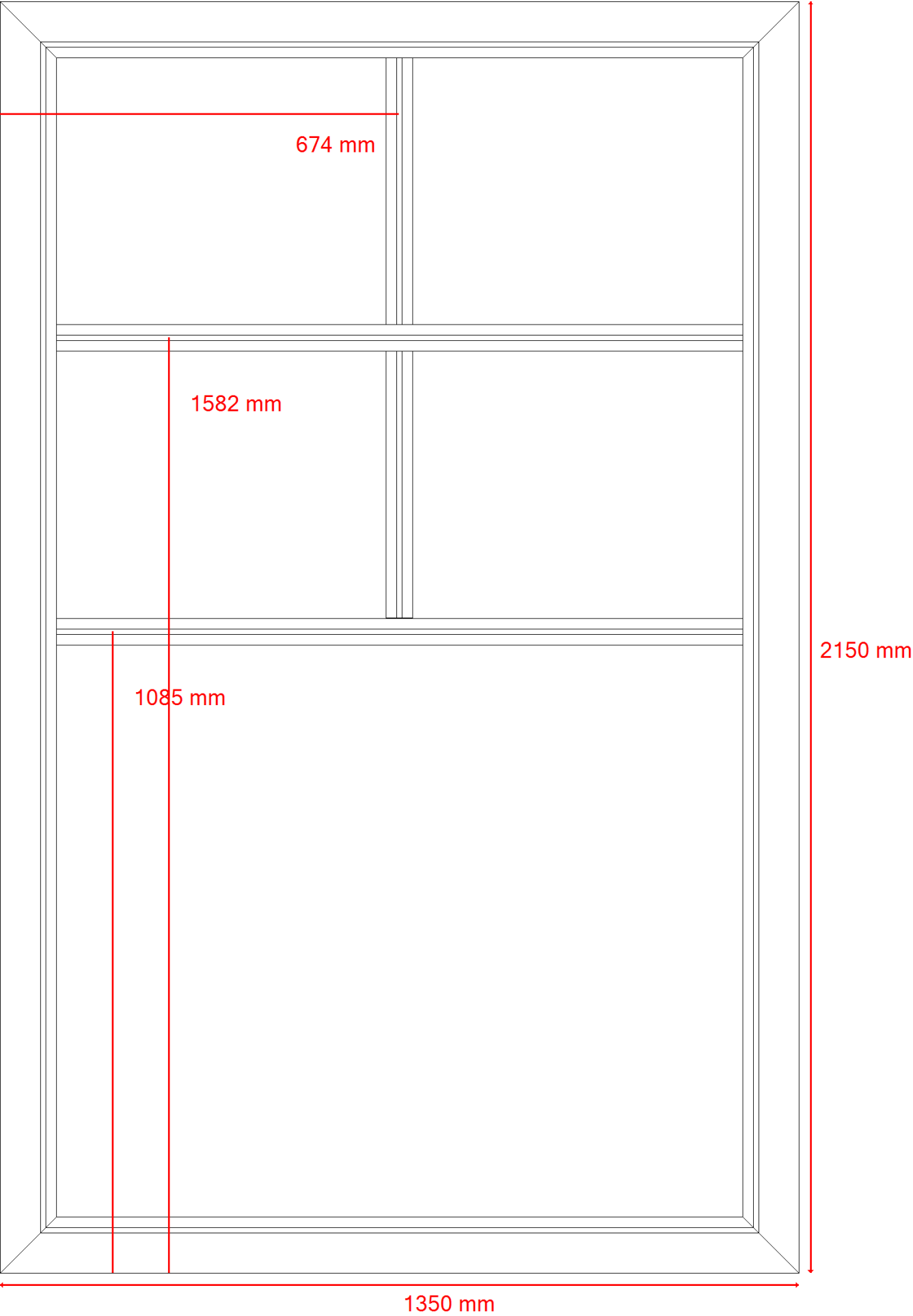
Werktekening incl. bematingen
