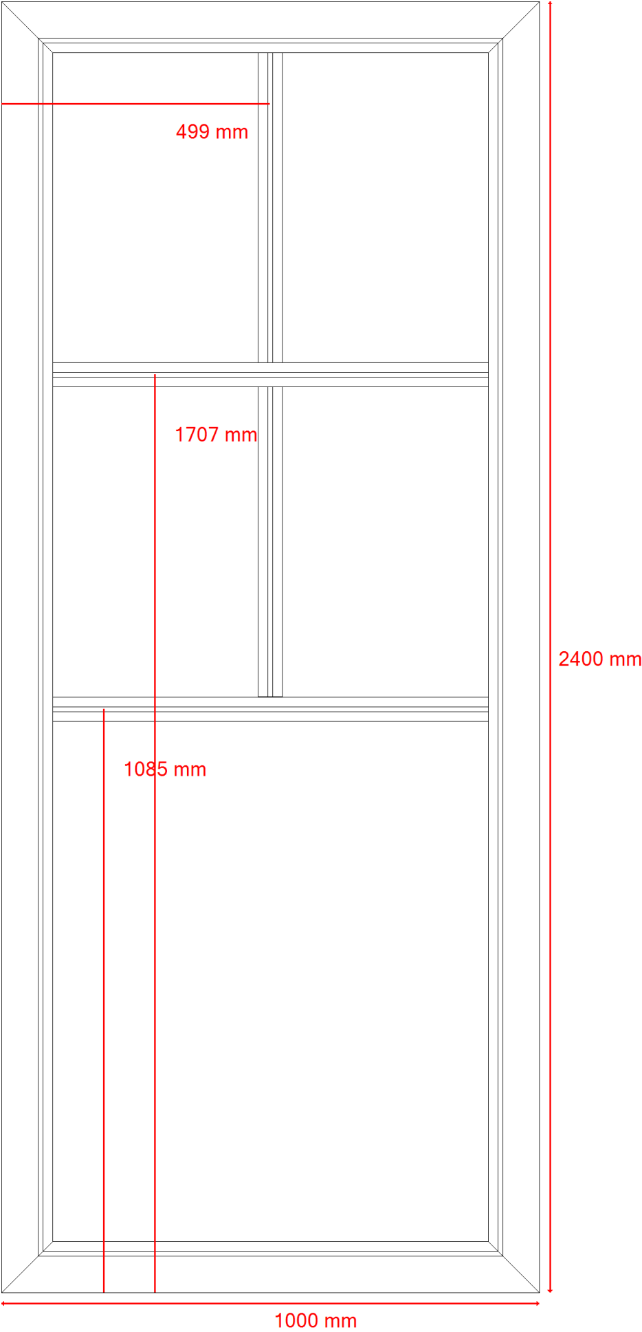
Werktekening incl. bematingen
