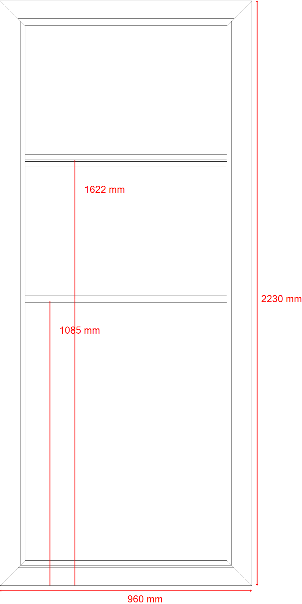
Werktekening incl. bematingen
