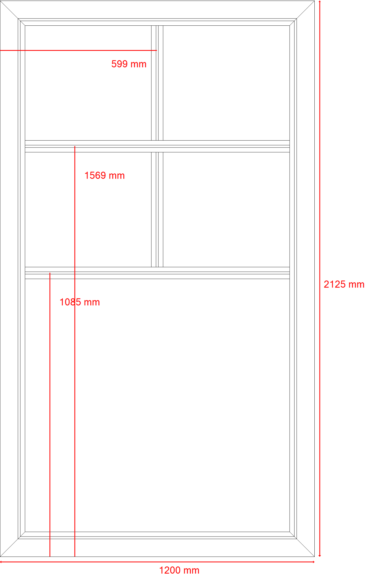
Werktekening incl. bematingen
