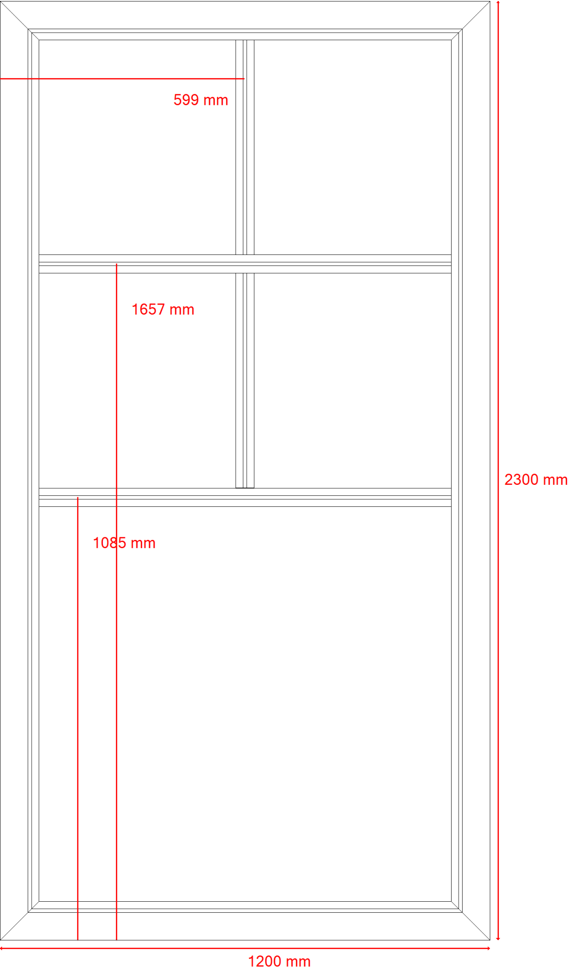
Werktekening incl. bematingen
