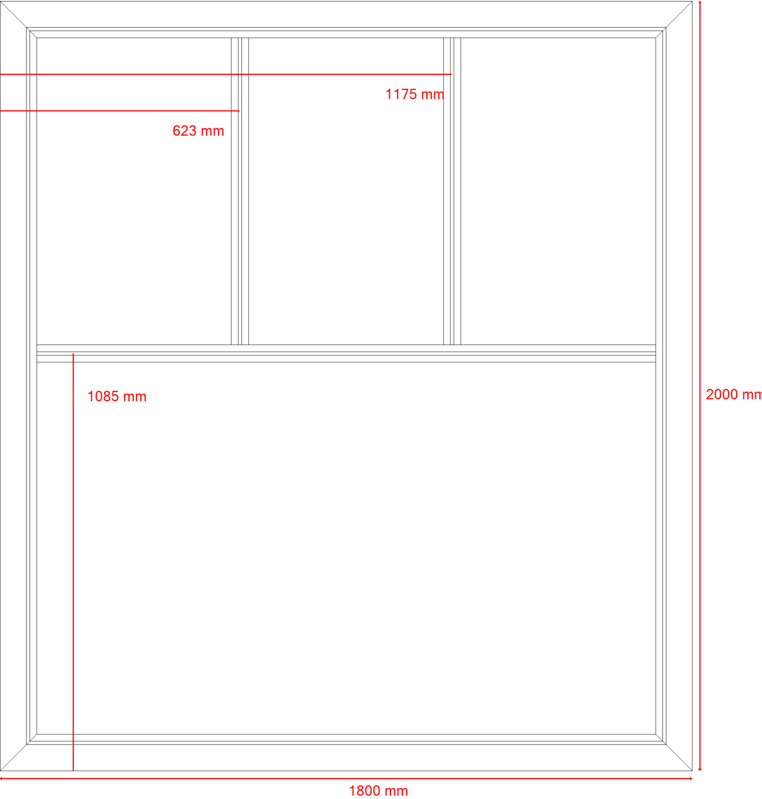
Werktekening incl. bematingen
